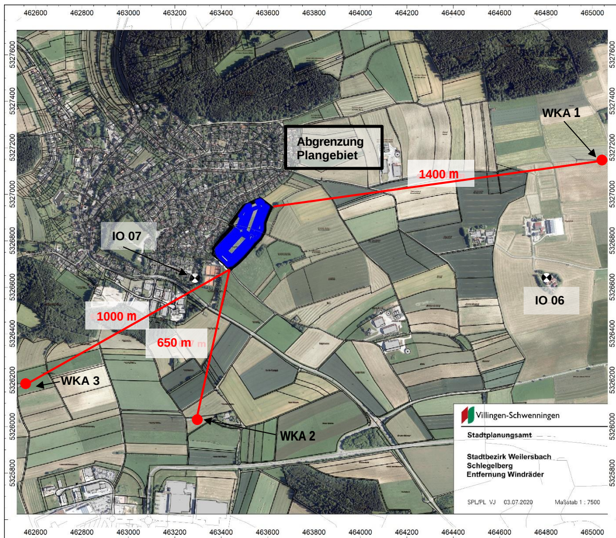
Abbildung 3: Lage der Windkraftanlagen und der maßbeglichen Immissionsorte. Plan-grundlage: /18/
