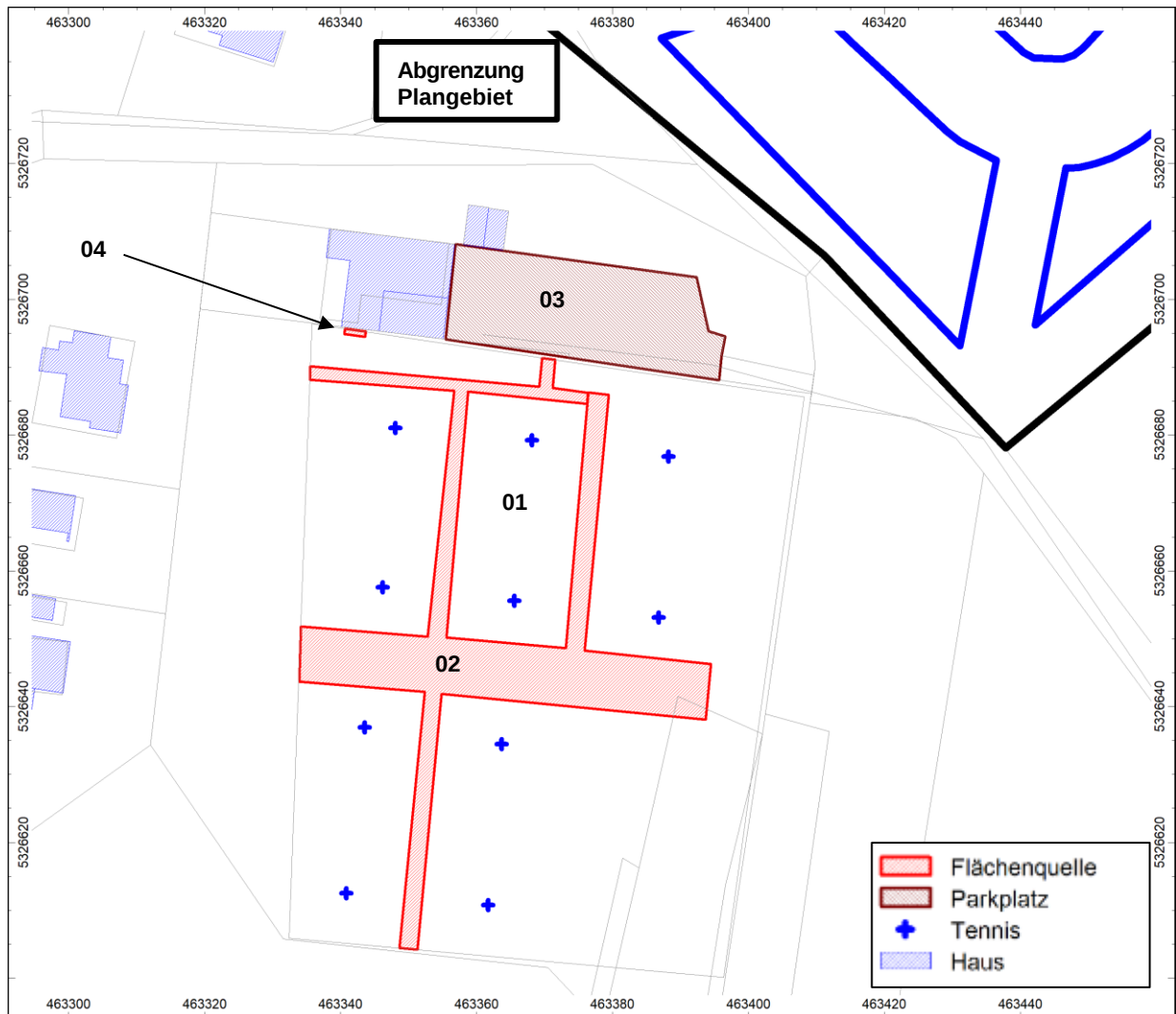
Abbildung 2: Lage der Schallquellen der Sportanlage
