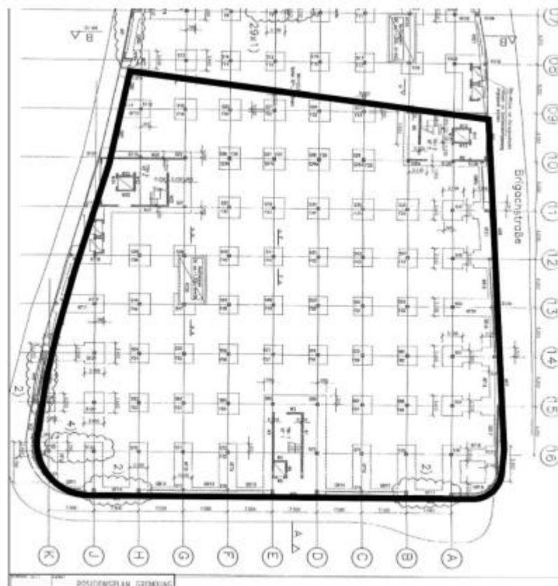
Abbildung 1: Ausschnitt aus dem Positionsplan der Gründung aus der Baumaßnahme 2001 [U1]
