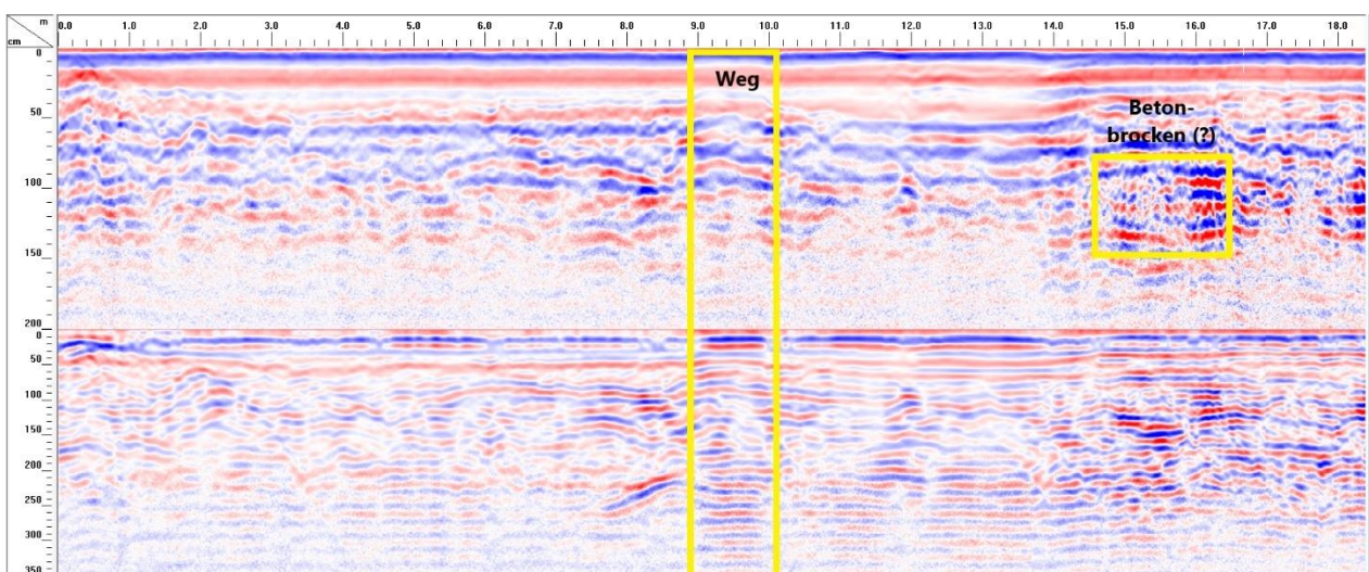
Abbildung 4: Radargramm entlang der Achse E (Ausschnitt) mit überlagerten Erläuterungen (oben: 800 MHz-Registrierung, unten: 300 MHz-Registrierung)
