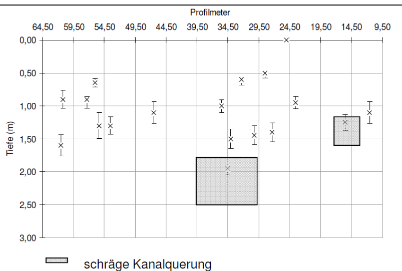
Abbildung 7: EMR-Sektion (Radargramm) entlang einer Straße (oben) sowie Darstellung einer integrativen Interpretation von mehreren EMR-Sektionen bzgl. querender Leitungen (unten). Zusätzlich zur interpretierten Tiefenlage der Oberkante der Leitungen (→ X) ist der jeweilige vertikale Schwankungsbereich eingetragen.
