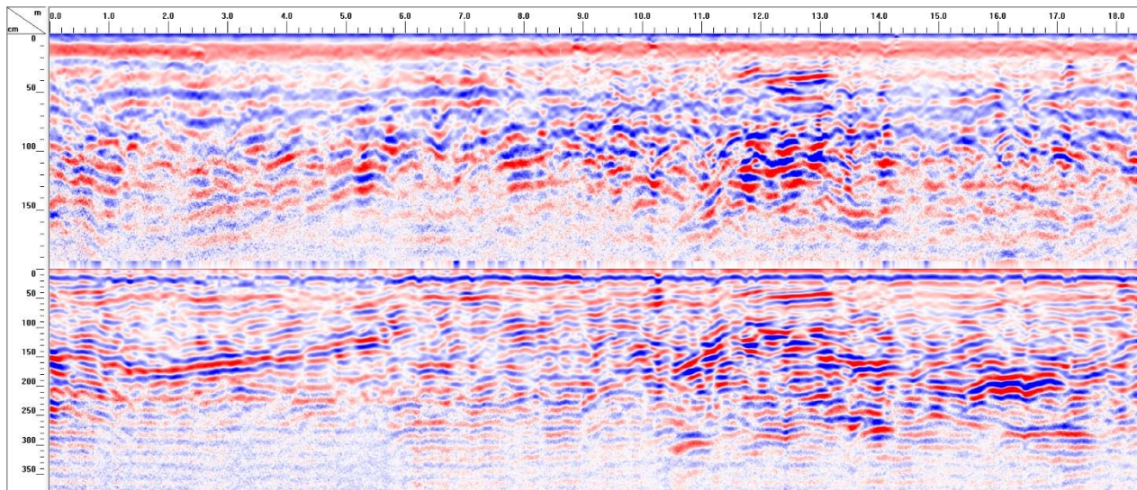
Abbildung 5: Radargramm entlang der Achse 11 (Ausschnitt; oben: 800 MHz-Registrierung, unten: 300 MHz-Registrierung)
