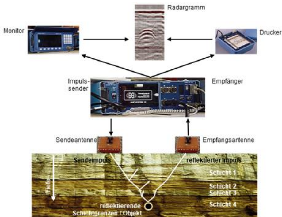
Abbildung 6 Schemabild der Funktionsweise des Georadars
