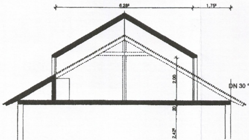
Systemskizze "Laternengeschoß"
